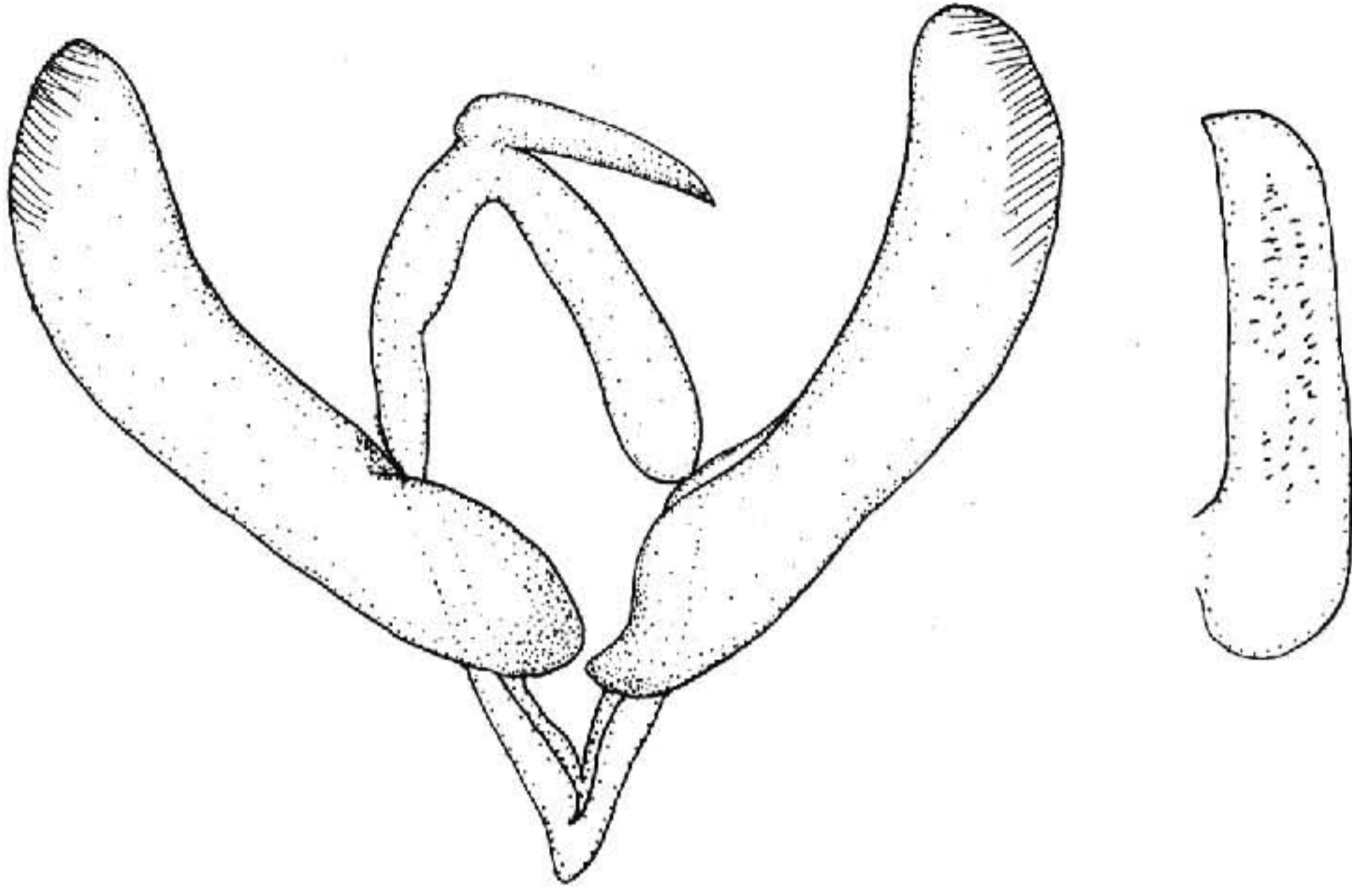
图 54 毛首夜蛾 Craniophora inquieta Draudt ♂ 外生殖器
