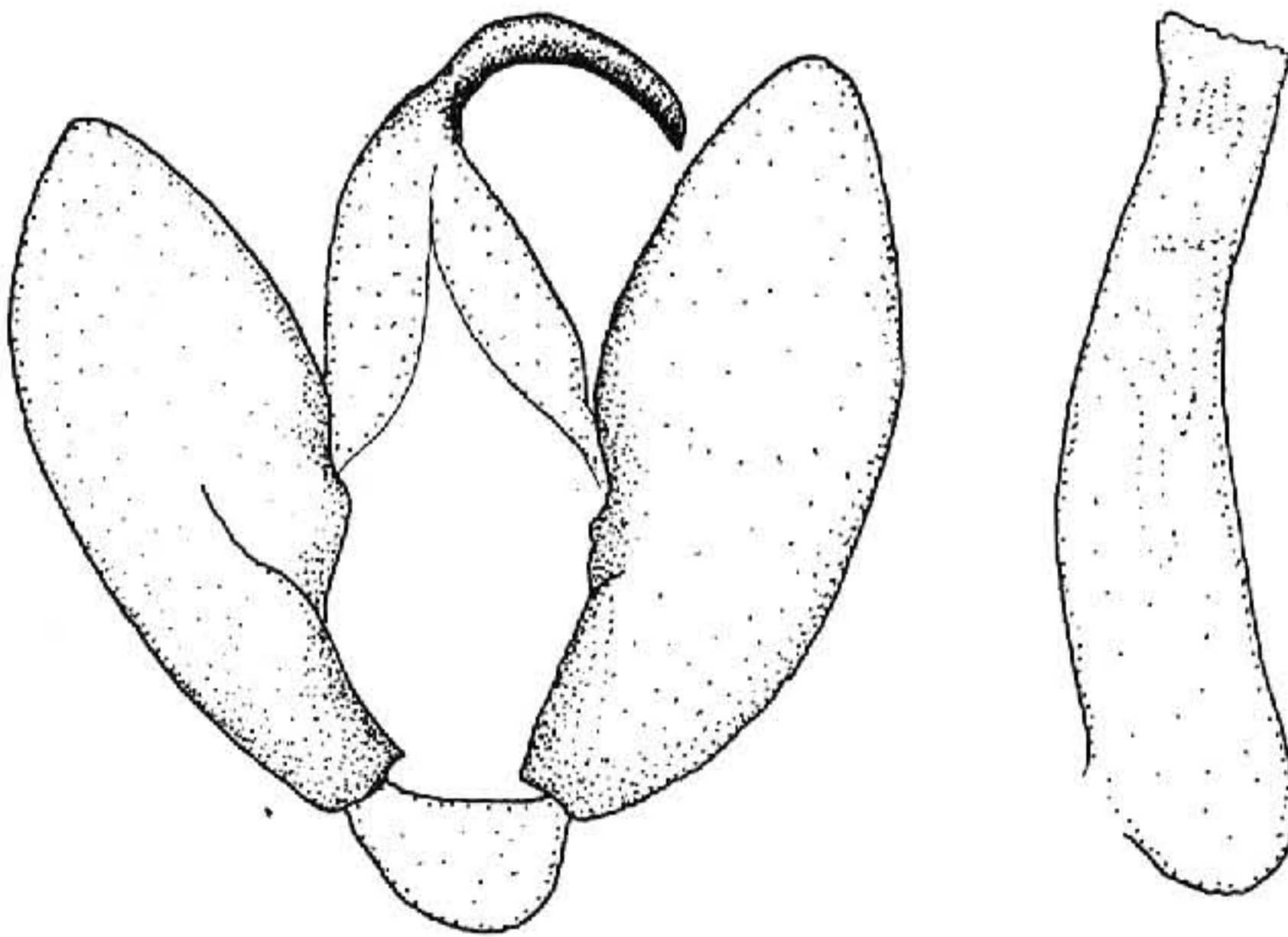
图 55 女贞首夜蛾 Craniophora ligustri (Denis et Schiffermüller) ♂ 外生殖器
